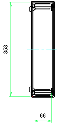
A-A (1:6)
